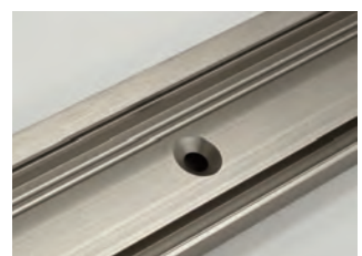
Eine saubere Rasterbohrung im Abstand von ca. 300 mm ist Standard bei Deubl Alpha. Solche professionellen Details erleichen und beschleunigen die Montage ganz erheblich.
