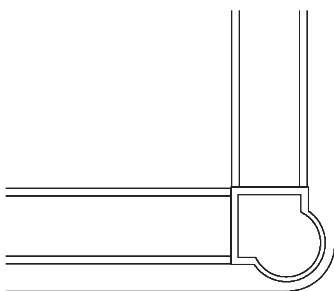
Tischplatte Rundercken Radius 25 mm
