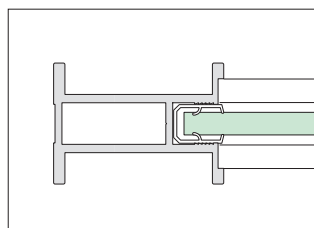
Profilquerschnitte
